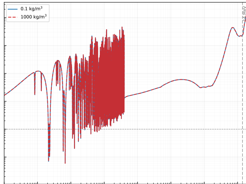
HCPB -- Th
